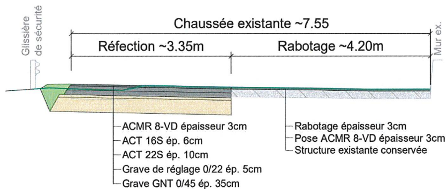
Figure 2 – Coupe-type remplacement du coffre de chaussée et rabotage
